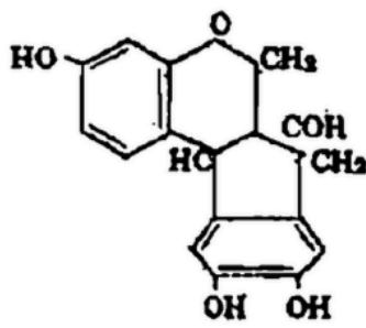
Brasilin
