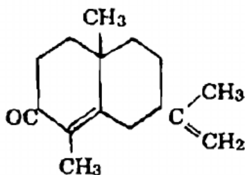
Cyperon
